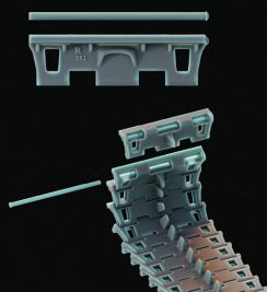
2 ГУСЕНИЧНЫЕ ЛЕНТЫ ПО 117 ТРАКОВ
